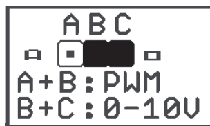
posición del jumper para enviar señales de 0-10 voltios
