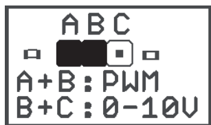
posición del jumper para enviar señales PWM
